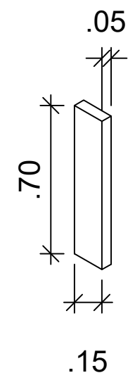
14 Perspectiva Madeira Divisória Cozinha/WC Esc.: 1/25
