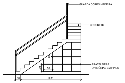
10 Escada Vista Lateral Esc.: 1/100
