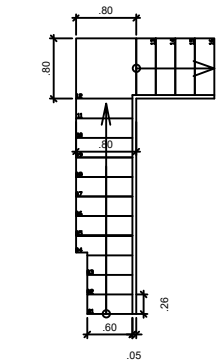
09 Escada Vista Superior Esc.: 1/100
