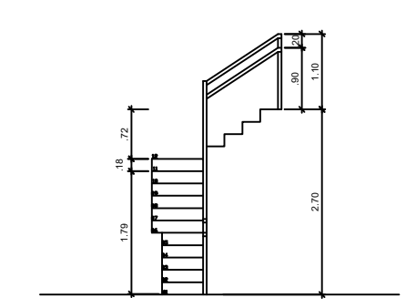
08 Escada Vista Frontal Esc.: 1/100
