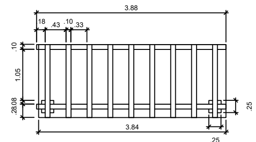
12 Pergolado Vista Superior Esc.: 1/75
