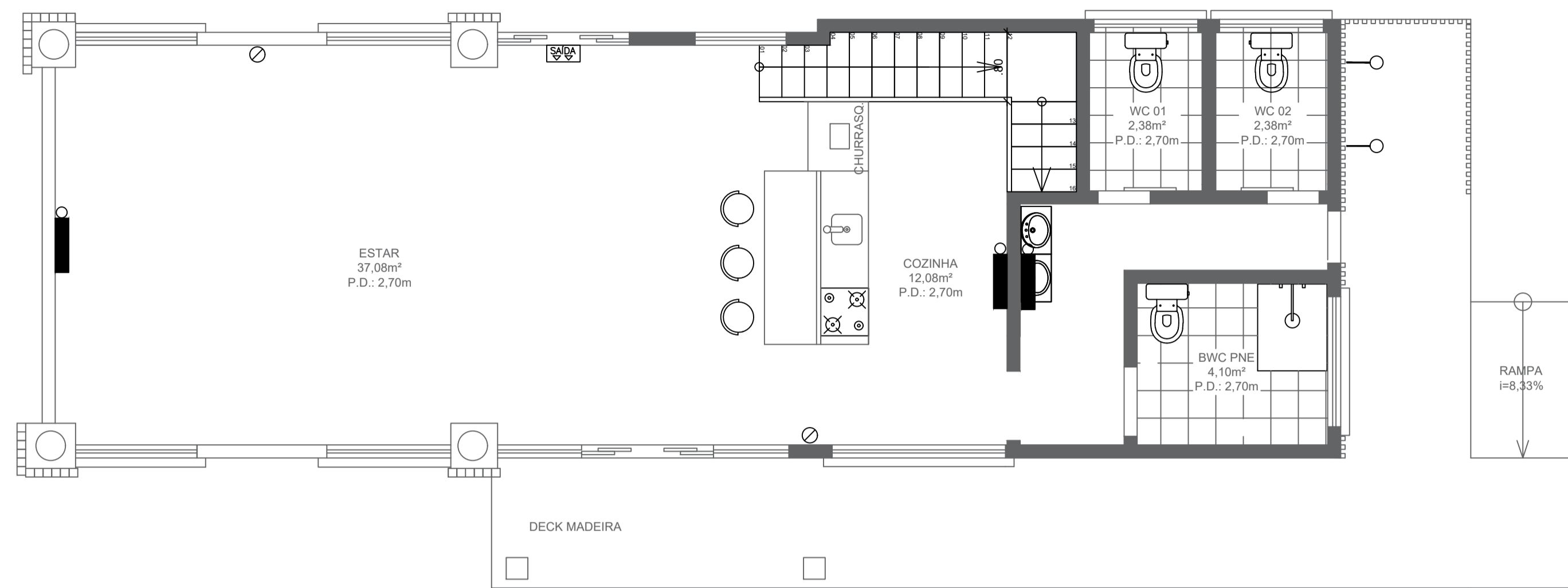
1 PLANTA BAIXA TÉRREO Escala: 1:50
