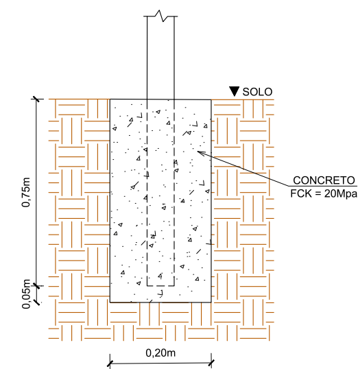
DETALHE DE FIXAÇÃO AO SOLO PARA PLACAS DE REGULAMENTAÇÃO E ADVERTÊNCIAS 0,80x0,20x0,20m
