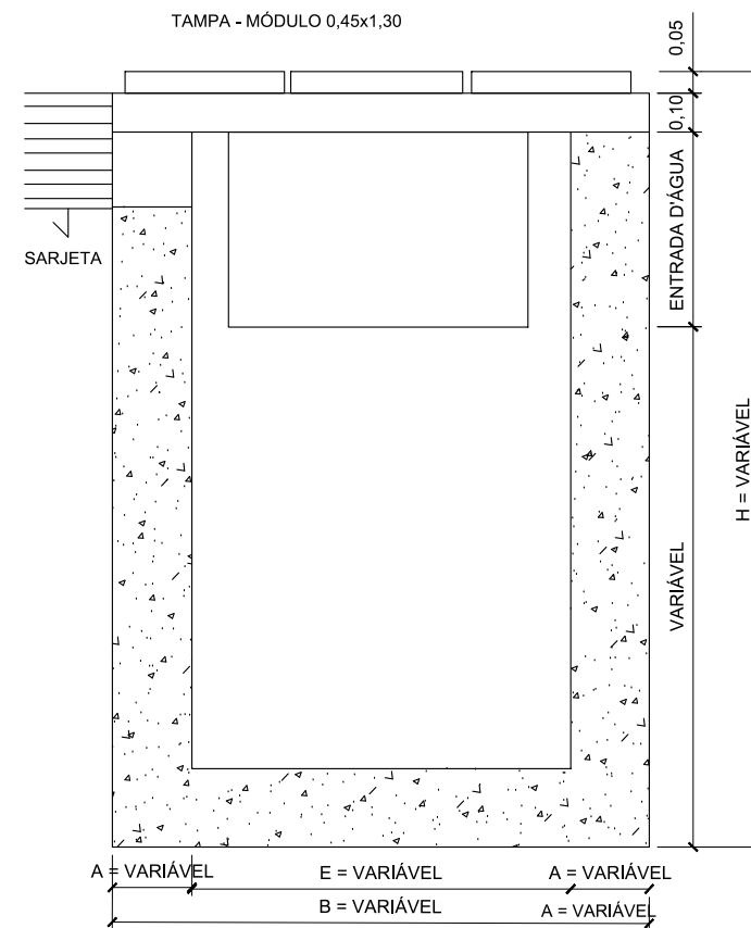
CORTE B-B'
