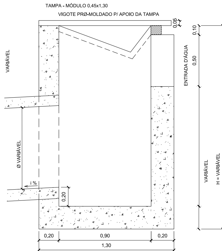
CORTE A-A
