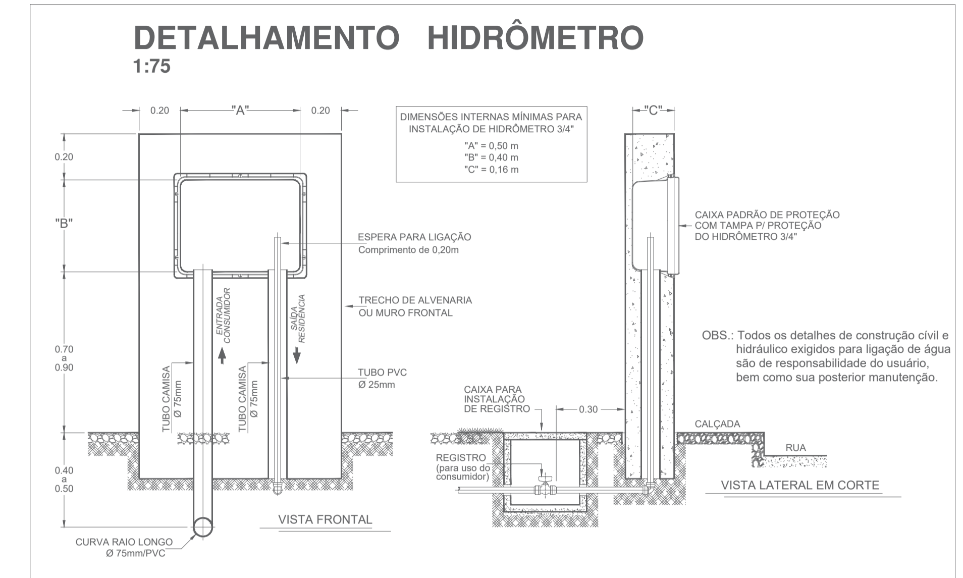
3 DETALHAMENTO HIDRÔMETRO Escala: 1:75
