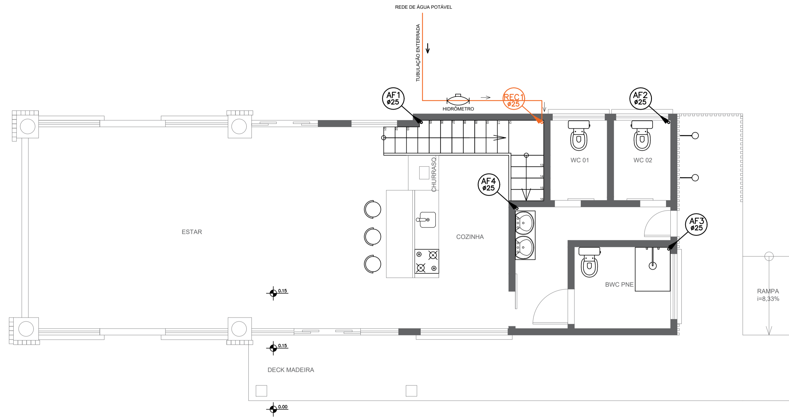
1 PLANTA BAIXA - Térreo Escala: 1:50
