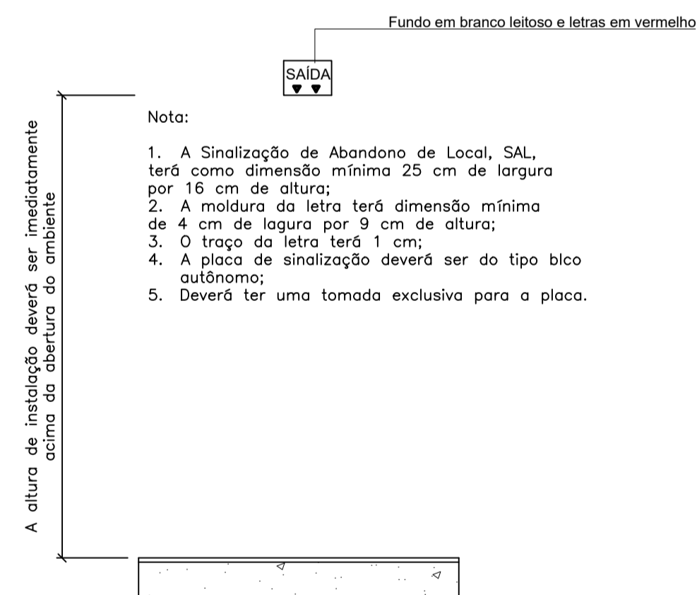
6 SINALIZAÇÃO S.A.L. Escala: 1:25
