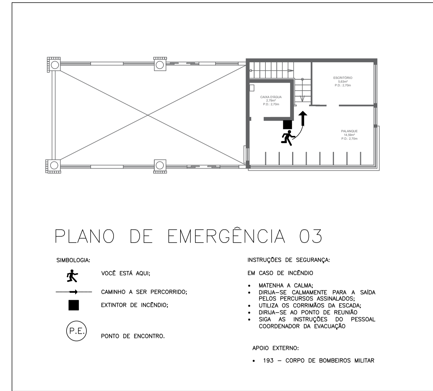
5 PLANO DE EMERGÊNCIA 03 Escala: 1:100
