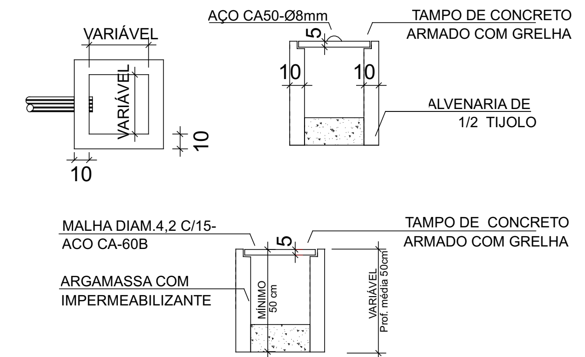
Detalhamento Caixa de Infiltração S/ Esc.
